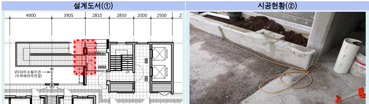
[그림 1] 동 출입구 경사로 계획 및 시공현황
